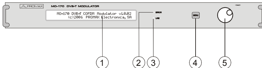
Figura 1.- Panel frontal.
